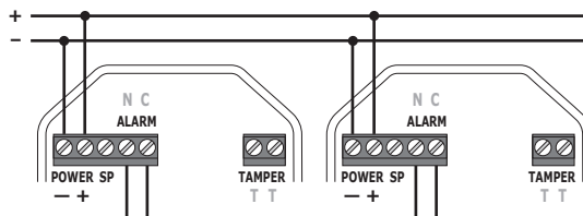
Conexión de varias sondas S1f.
